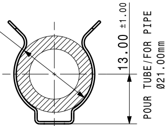
EXEMPLE D'UTILISATION / USE CONDITION ECHELLE / SCALE: 1:1
