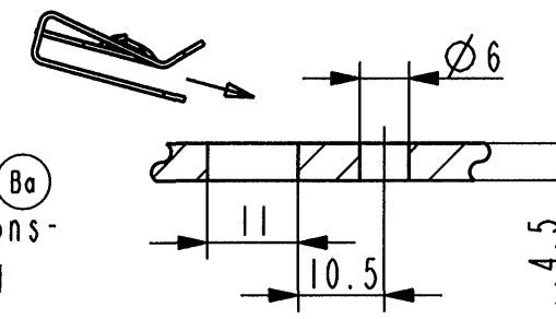
Einbausituation 1:1
