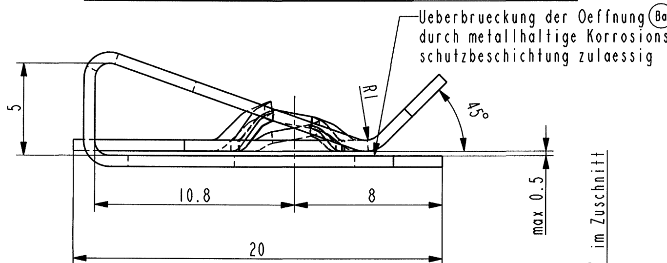
Einbausituation 1:1
